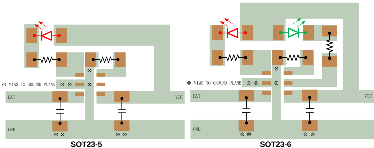
图9 推荐PCB 布局举例
