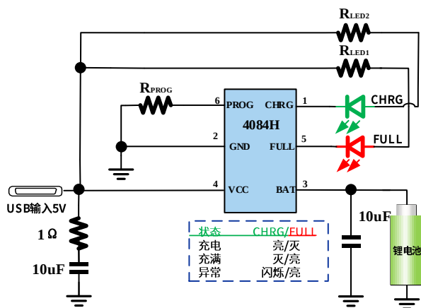
图 1 LGS4084HB6 典型应用拓扑
