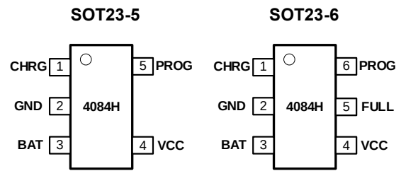
图 3. 引脚排列
