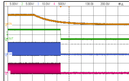
图 5.2-16 5V Output EN Power Off
