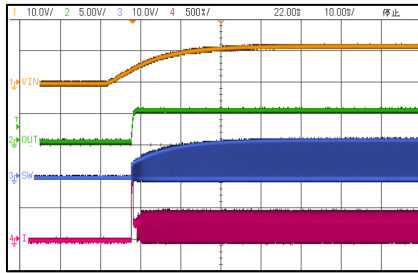
图 5.2-13 5V Output VIN Power On
