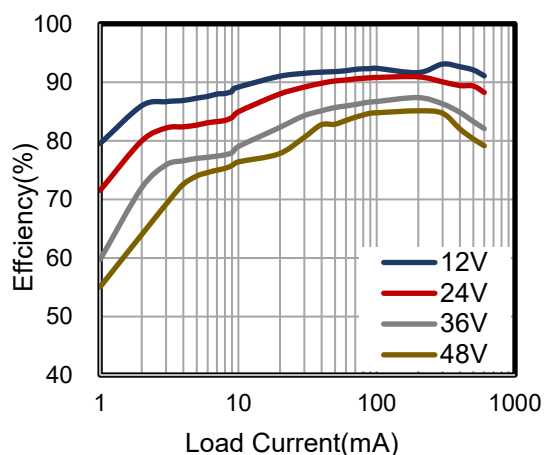
图 5.2-2 Efficiency 5V Output
