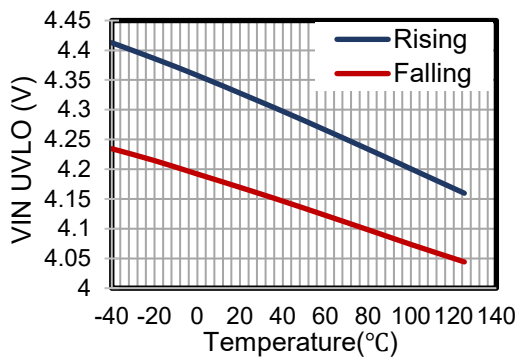
图 5.1-3 VIN UVLO
