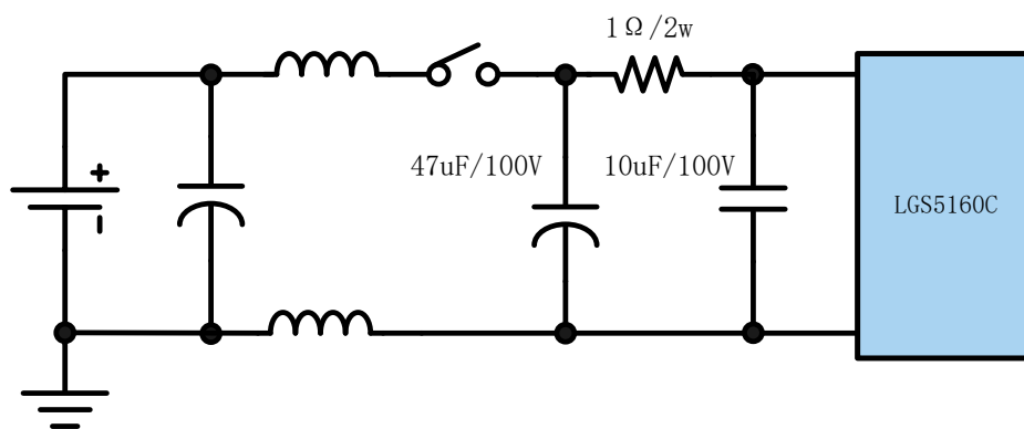
Figure 26 b. 单电阻滤波电路情况下热插拔示意图
