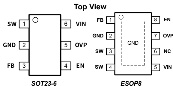
图 3.1 封装与引脚排列
